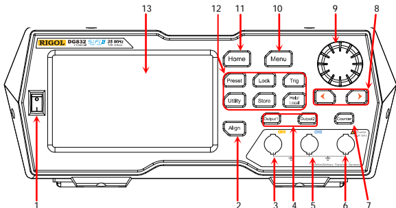
图 1 前面板
