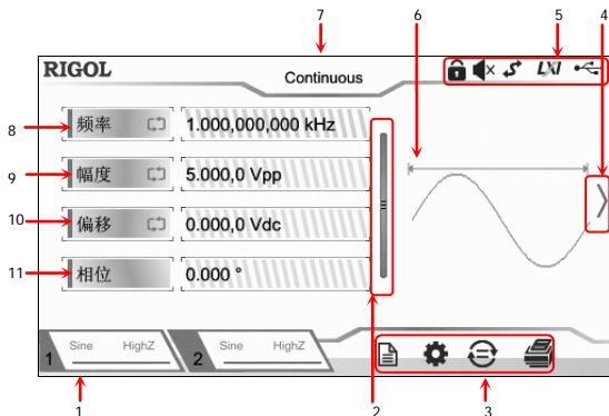
图 3 用户界面
