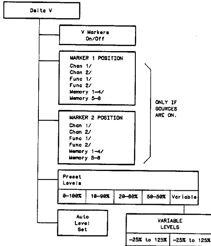
Figure 8-1. Delta V Menu.
