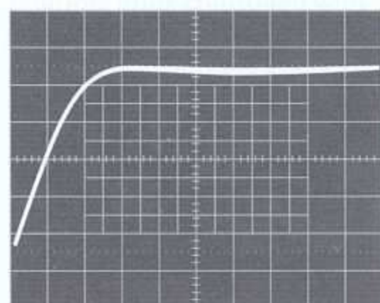
Actual 228A transient response, 100V range @ 1A. Vert.: 20V/div. Horiz.: 0.2ms/div.
